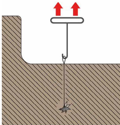
Anker verriegeln (Installationshinweise Pkt.3)
